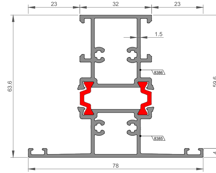
FS-2321 Kanat İçi Orta Kayıt Profili Mullion Profile for Sash
