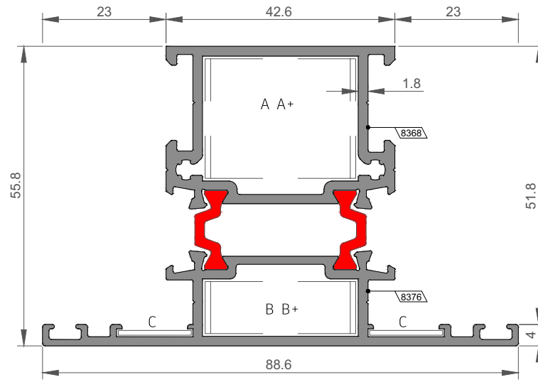
FS-2132 Orta Kayıt Profili Mullion Profile
