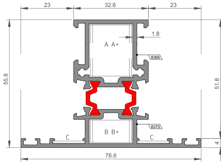
FS-2131 Orta Kayıt Profili Mullion Profile
