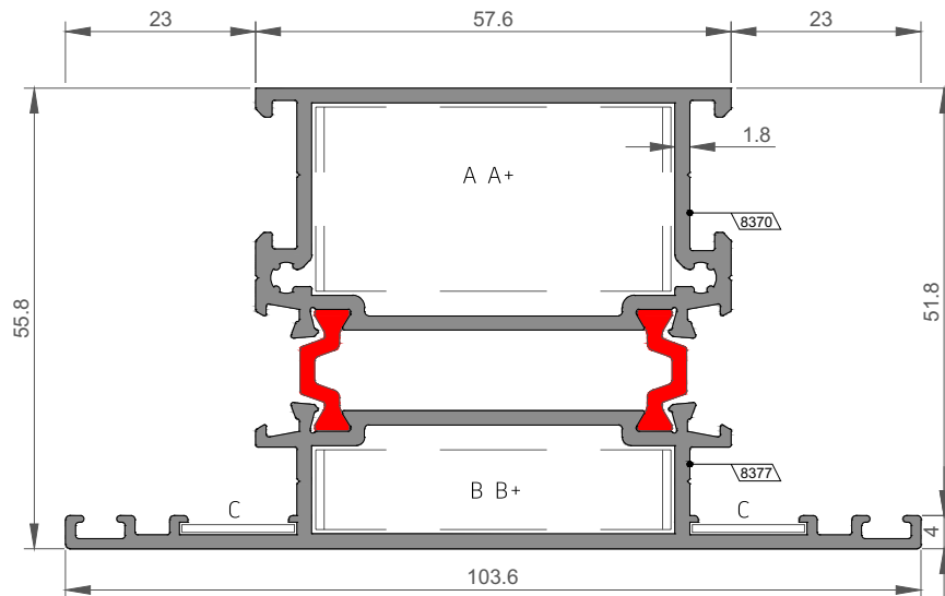
FS-2133 Orta Kayıt Profili Mullion Profile
