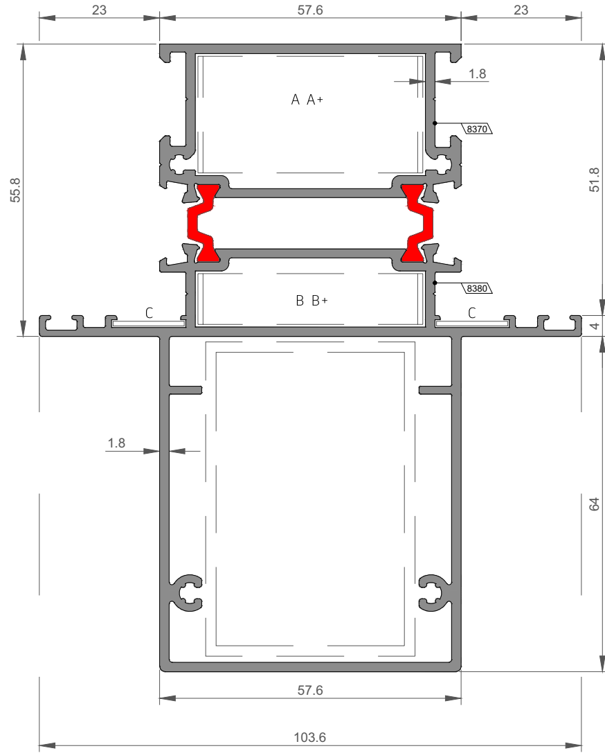
FS-2233 Takviyeli Orta Kayıt Profili Reinforced Mullion Profile
